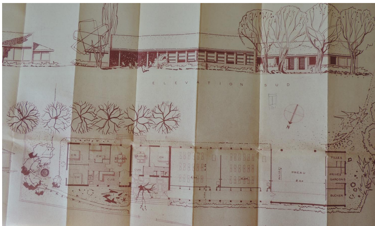
Élévation sud et plan, M. Dosse et associés, 1955 (AC Fareins. M1).
