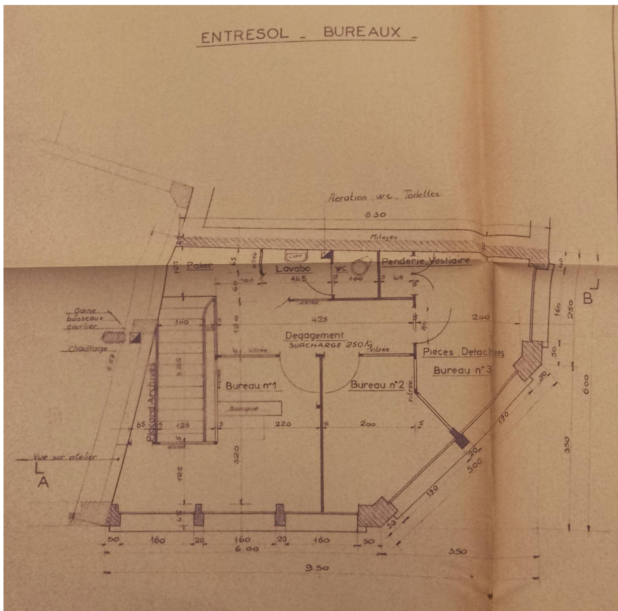
Plan de l'entresol (bureaux)
