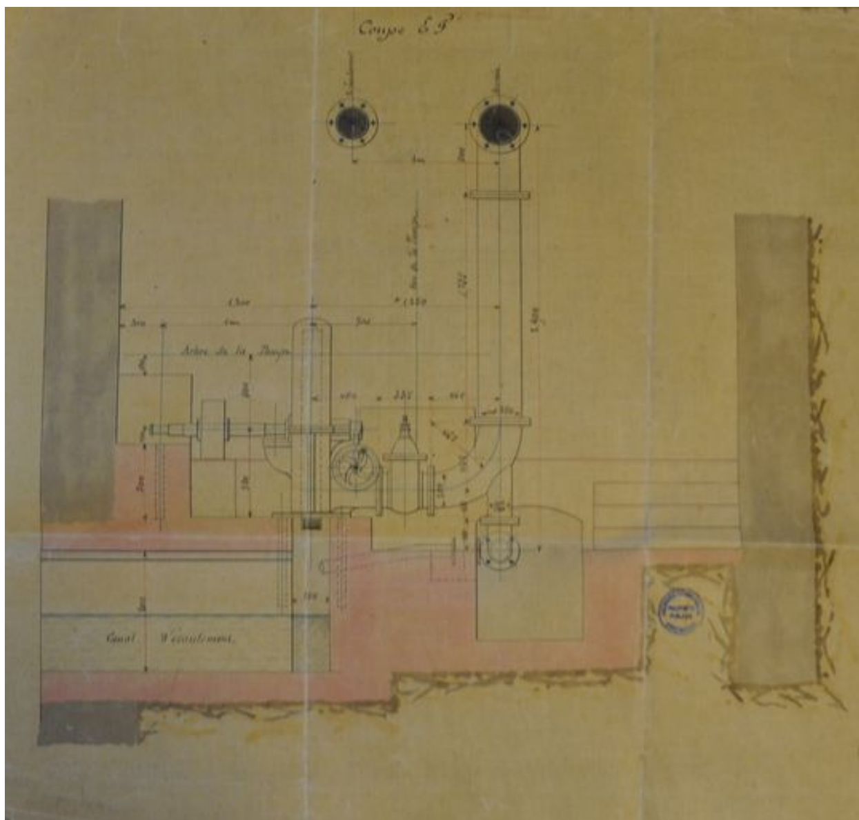
Coupe E.F. Plan. Archives municipales d'Annemasse © Archives municipales d'Annemasse. 36/36
