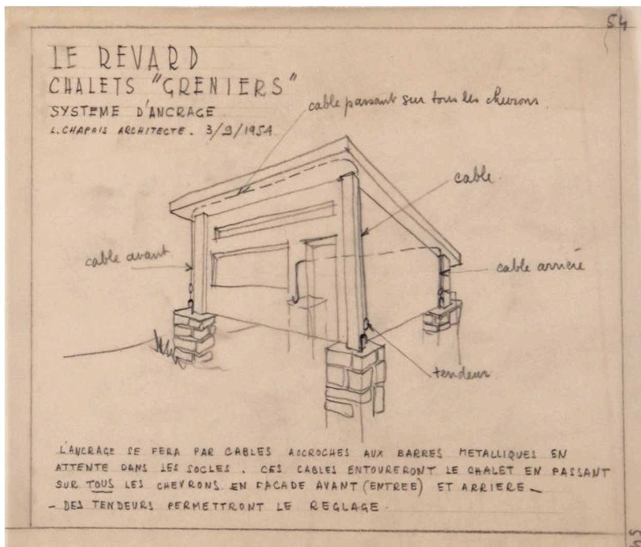
Système de câbles pour tenir la toiture, 1954
