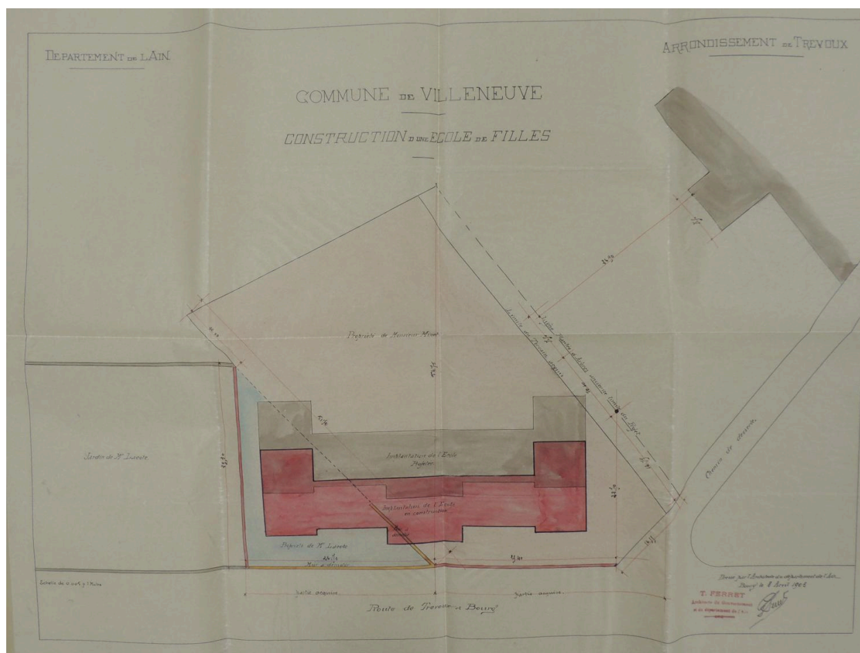
Plan d'ensemble, T. Ferret 1903 (AD de l'Ain. 2 O Villeneuve 5).
