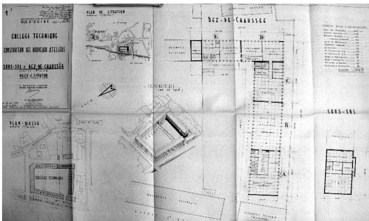
Collège Technique Plan du sous-sol, rez-de-chaussée, masse et situation, Projet, A. Bugnard 8 octobre 1960 (AD Savoie, 1350 W 615)
