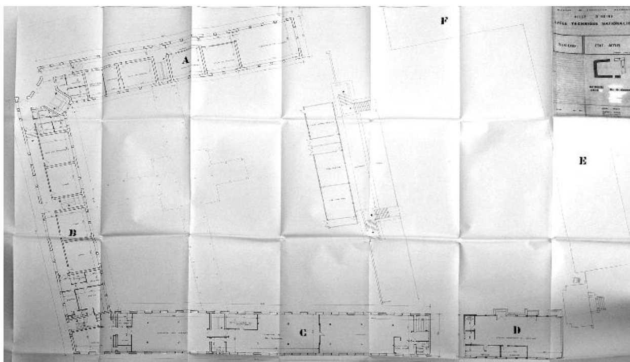
Lycée Technique Nationalisé, Plan bâtiments A, B, C et D rez-de-chaussée, A. Profit Mai 1974 (AC Ugine, 6 W 106)
