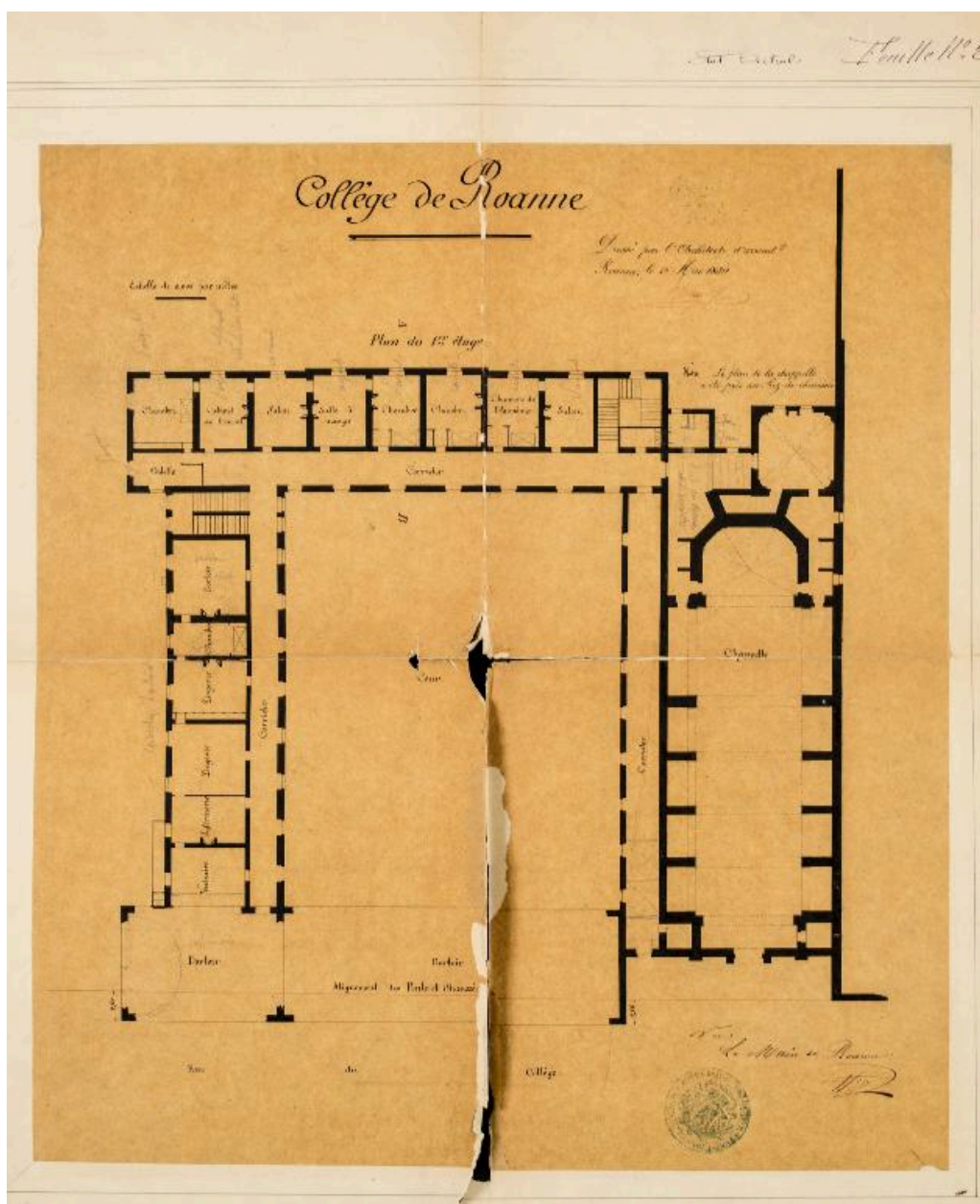
Plan. Feuille n°1. Plan du 1er étage. État actuel (10 mai 1880)
