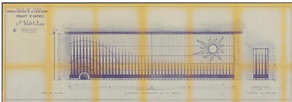
Grille et portillon : coupe et élévations, février 1968
