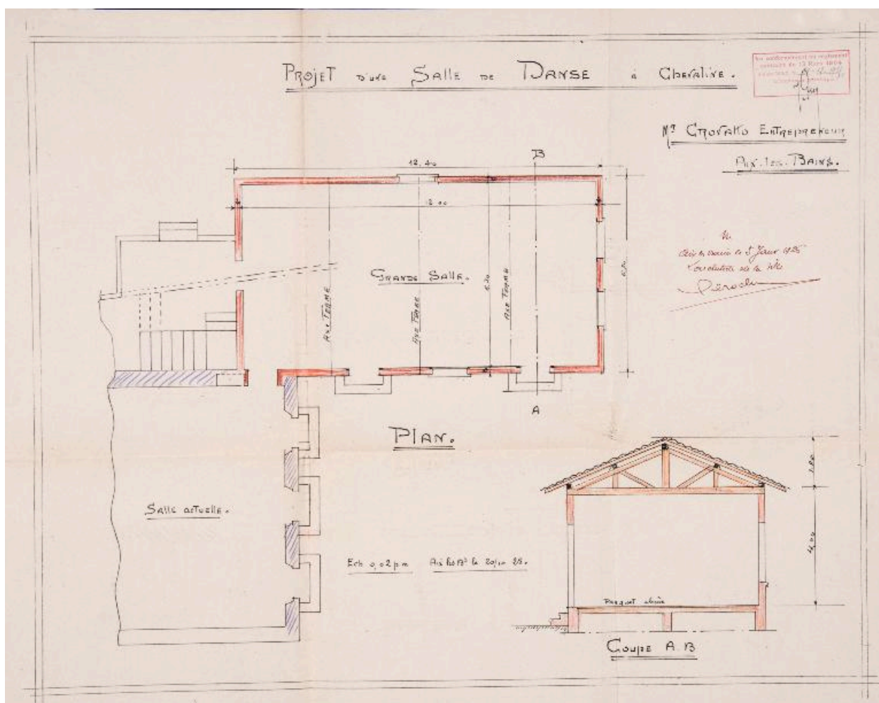
Projet d'une salle de danse : plan et coupe, 1925
