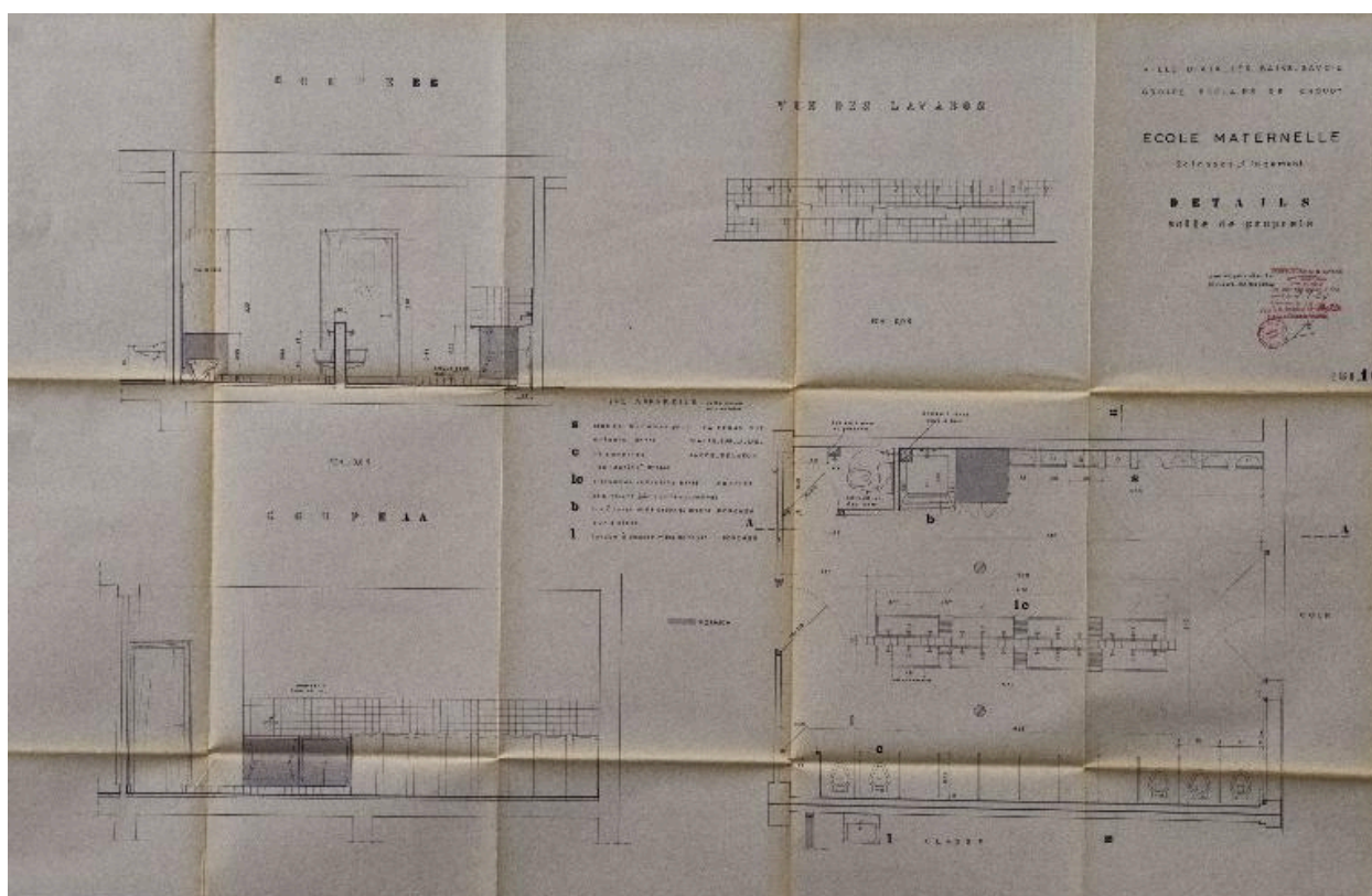
Sanitaires, plan, coupes et détails, 1966
