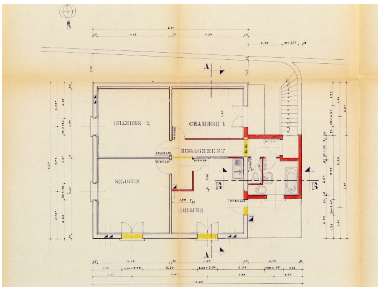
Plan, projet d'agrandissement
