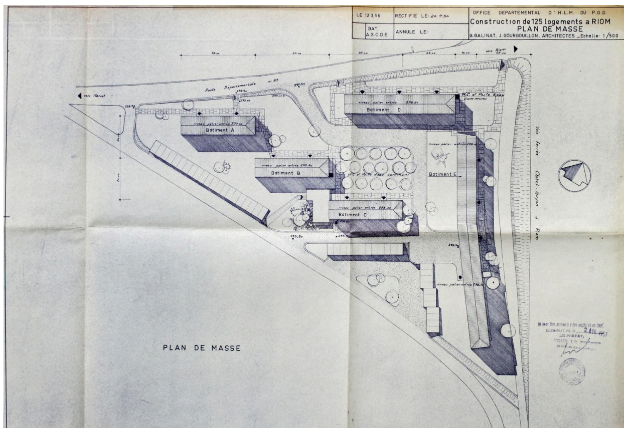
Riom, la cité HLM de la route de Marsat, plan de masse, 1956, G. Galinat et J. Gourguillon architectes (Archives municipales de Riom).
