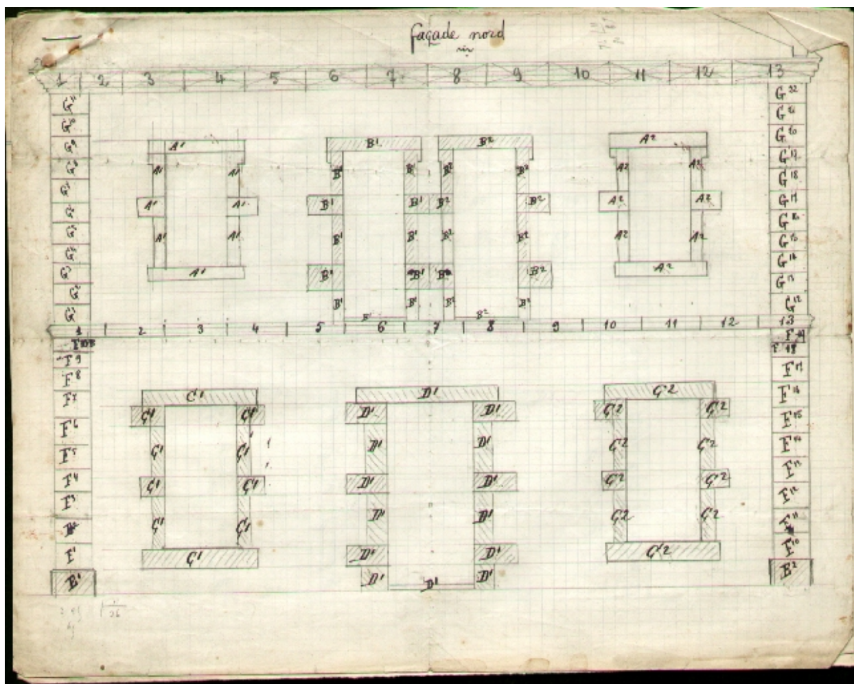
Elévation nord
