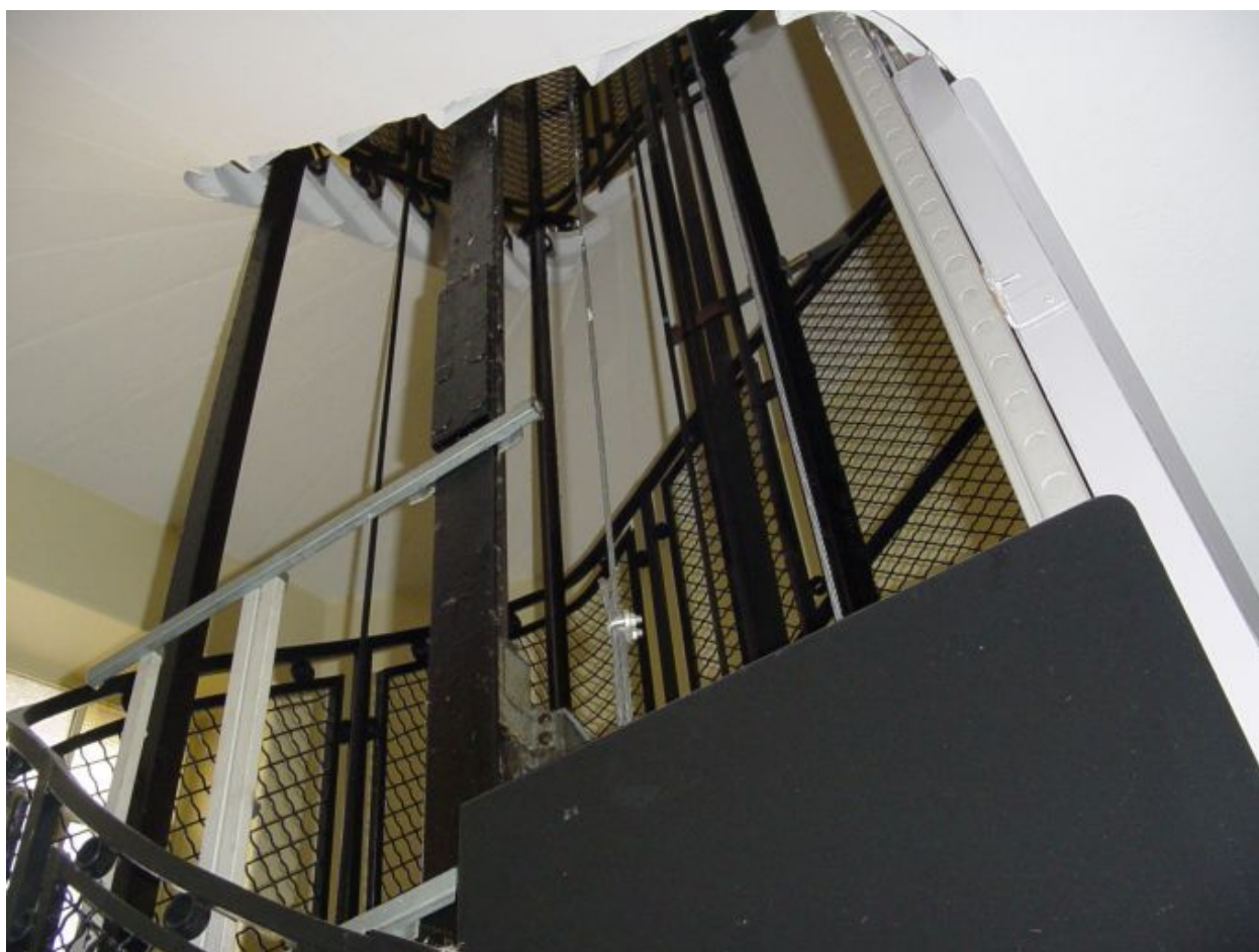
Cage d'ascenseur
