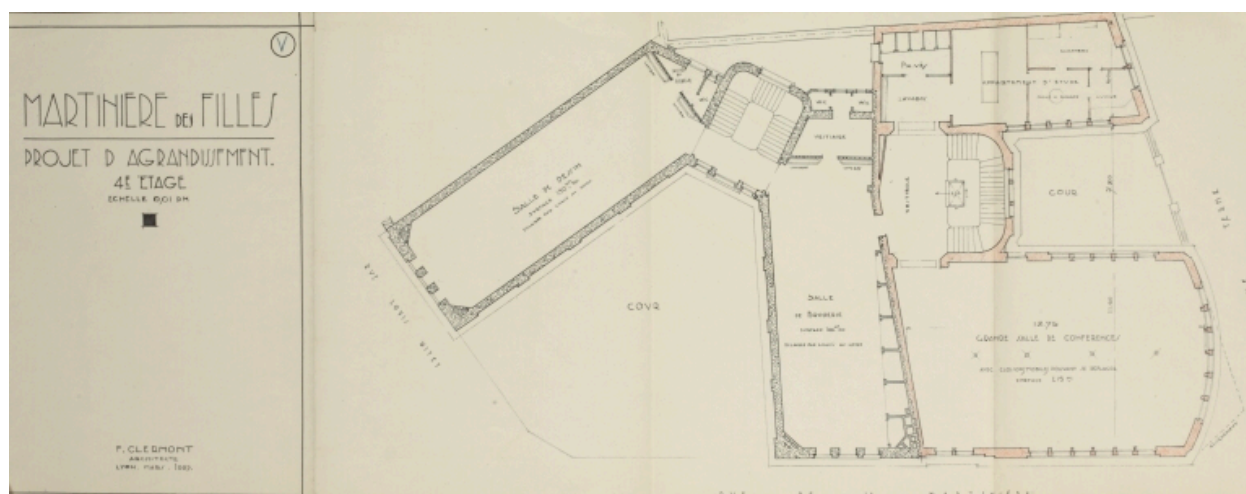
Agrandissement. 4ème étage, 1:100. François Clermont. Mars 1929. Document figuré. Papier 40 x 75 cm. Fondation Martin. non coté
