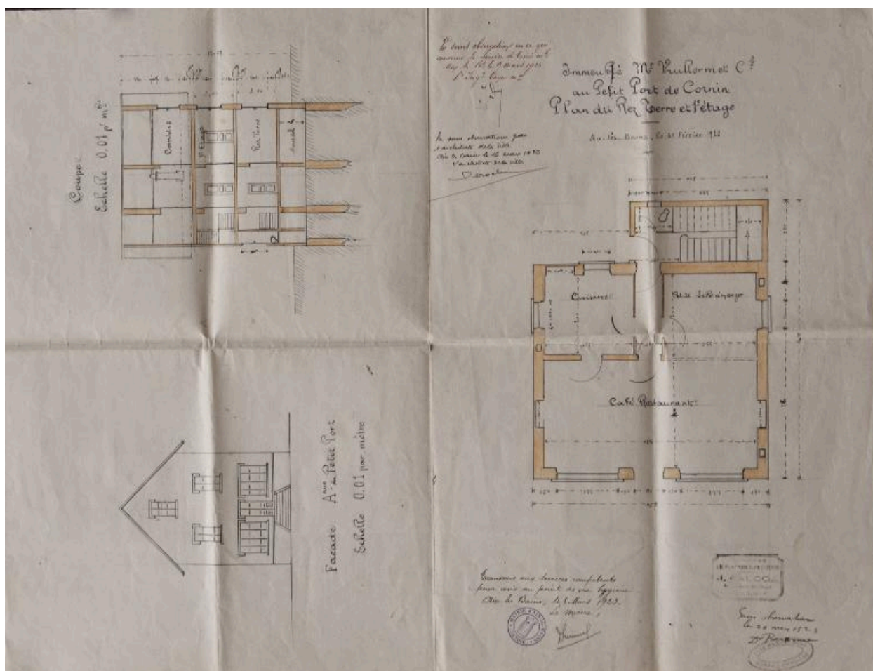
Hôtel Petit Charmant, 1923 : plan, façade et coupe
