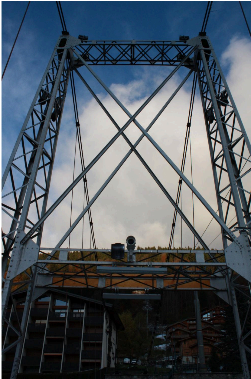
Passerelle François-Baud Grand-Hotel, détails haubans
