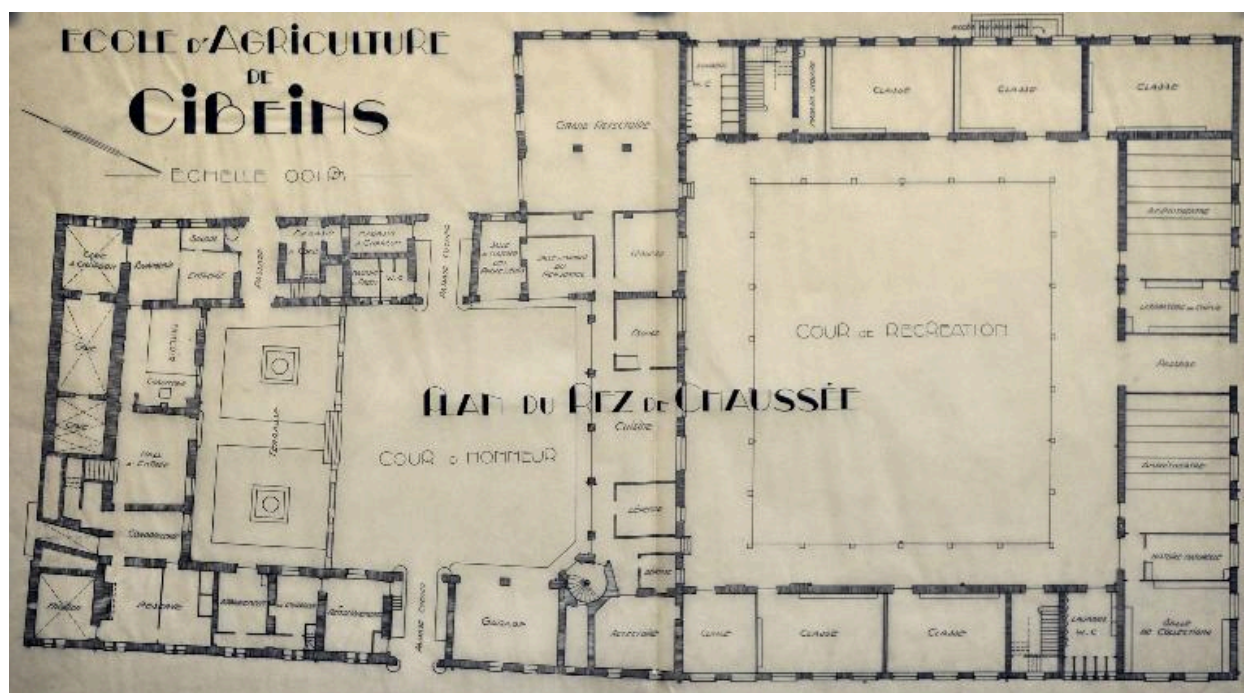
Projet d'aménagement du château par Ch. Meysson, ca 1920 : plan du rez-de-chaussée (AC Lyon, 111 WP 028)
