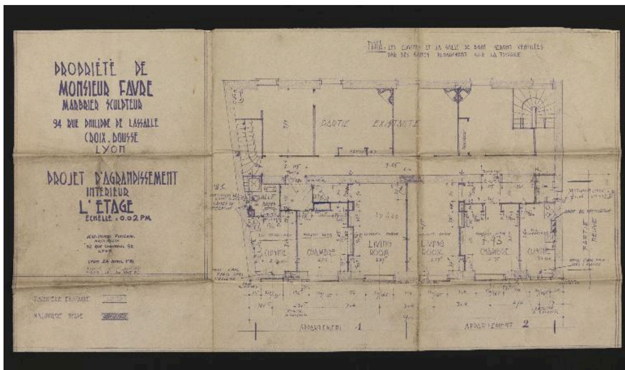
Plan de l'étage : projet d'agrandissement intérieur, Jean-Pierre Fonterme architecte, 24 avril 1951
