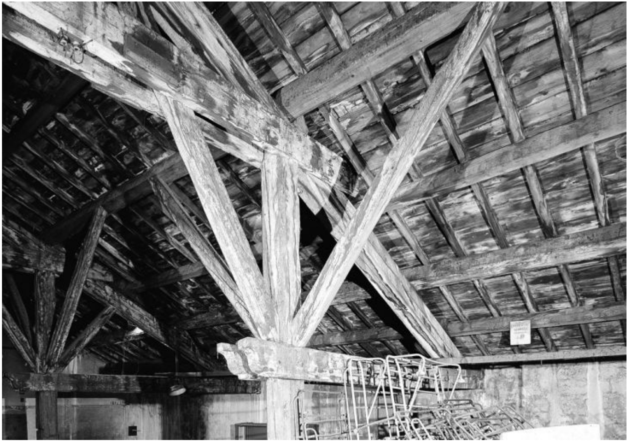
Détail de la charpente du fenil
