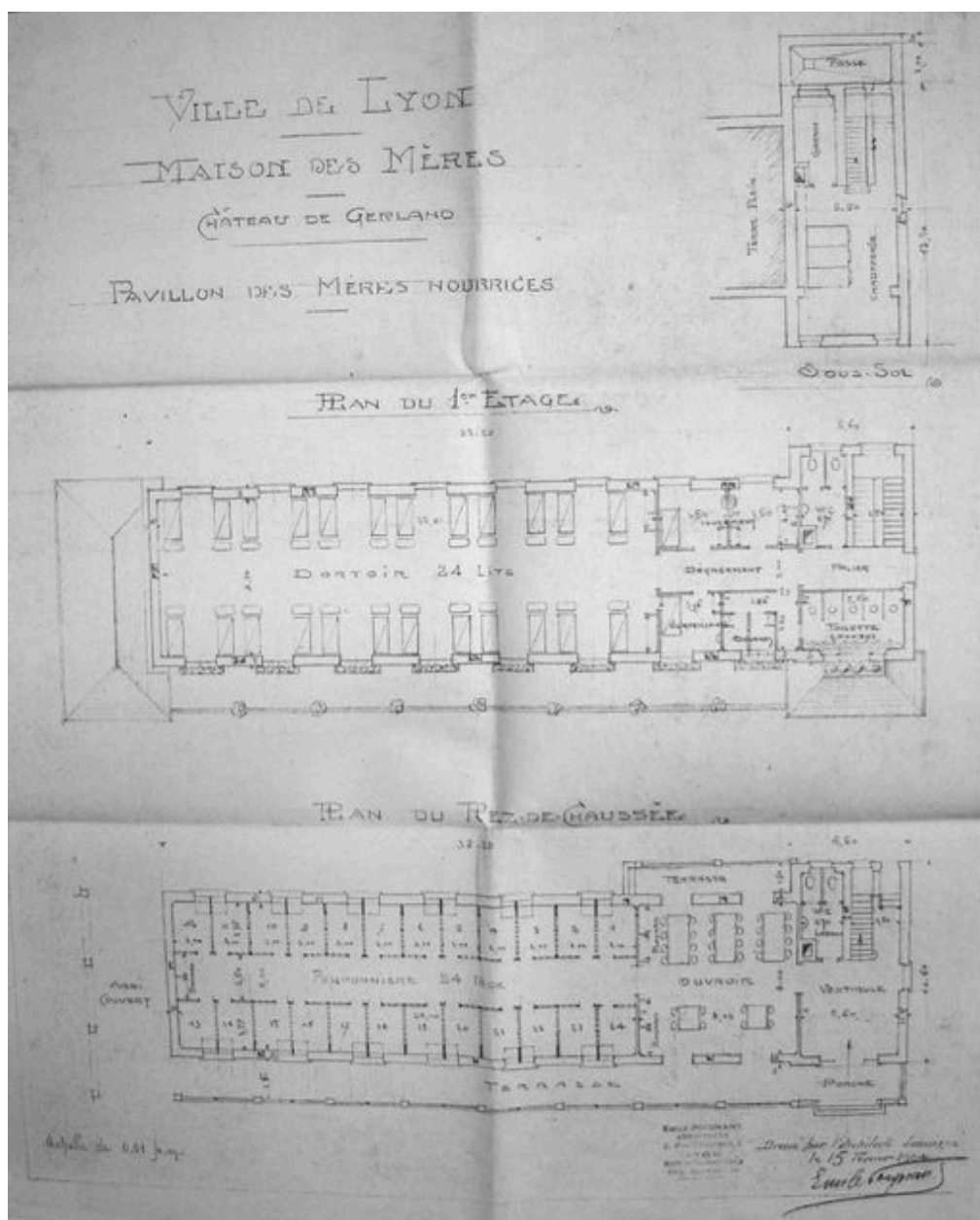
Pavillon des mères nourrices : plan du rez-de-chaussée, plan du 1er étage, Emile Poignant architecte, 1924 (AC Lyon 1741 W 5)
