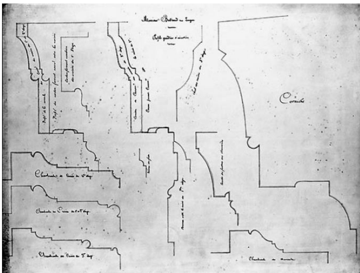
Feuille 23, Profils grandeur d'exécution, par H. Feuga, 1869
