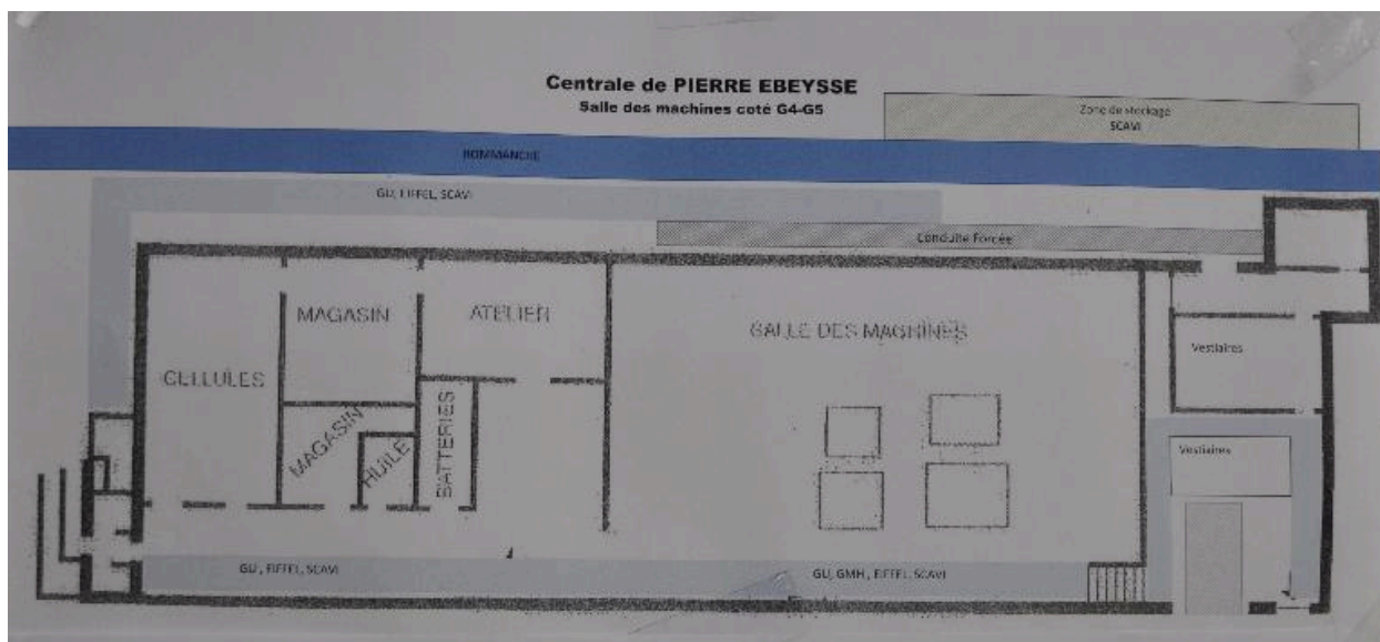
Plan de la salle des machines de la centrale Pierre-Eybesse
