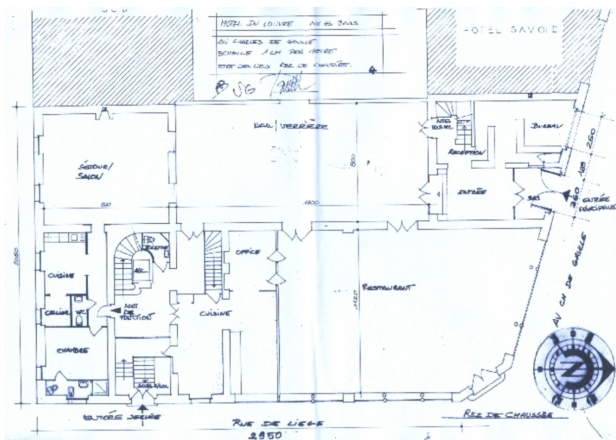
Plan du rez-de-chaussée avant travaux
