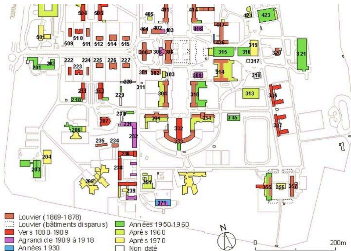
Plan-masse chronologique et localisation de l'ensemble des bâtiments, détail de la moitié sud
