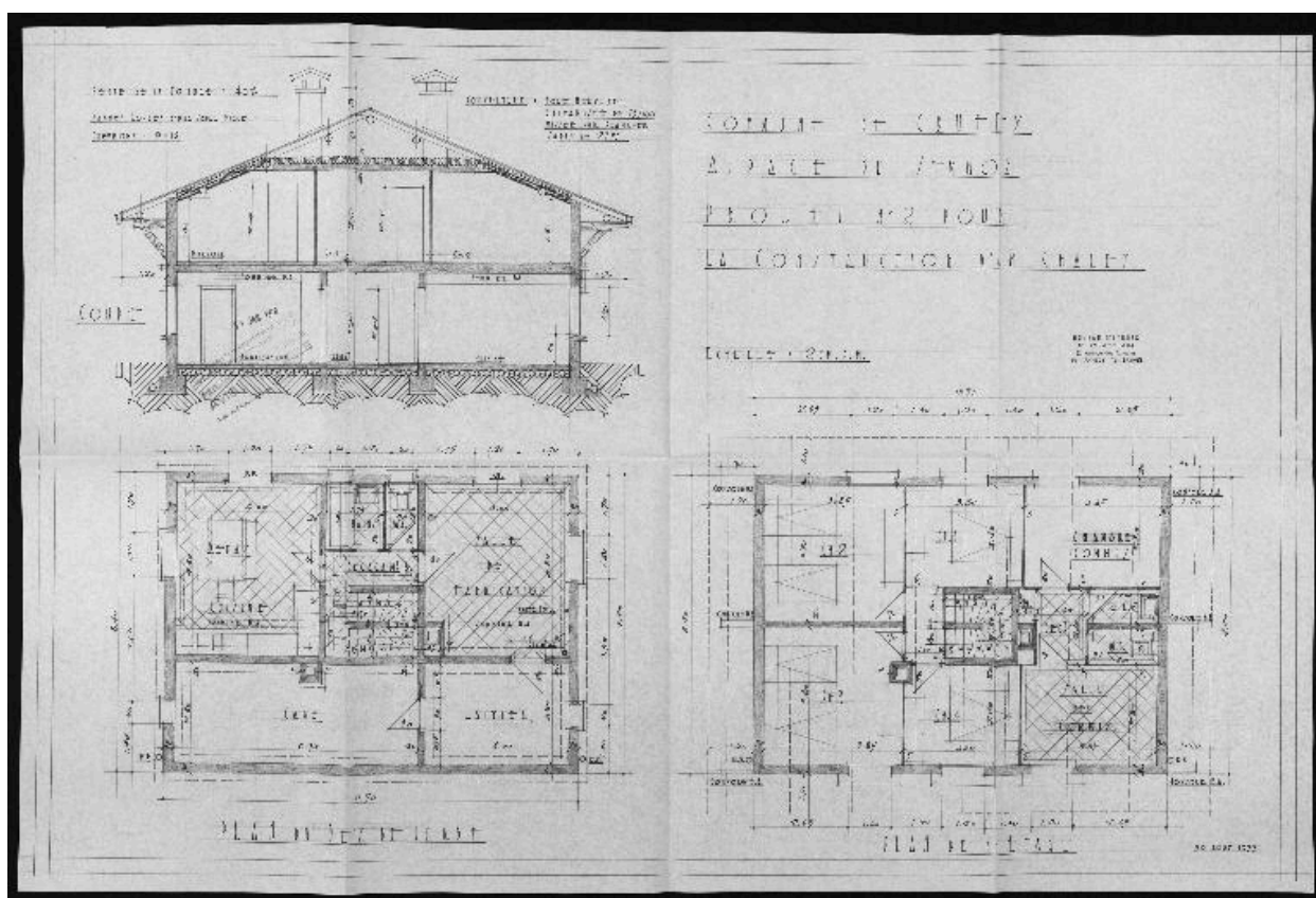
Commune de Gruffy. Alpage du Semnoz. Projet n°2 pour la construction d'un chalet. [2] Plan du rez de terre. Plan de l'étage. Coupe. 30 août 1977 (AC Gruffy).
