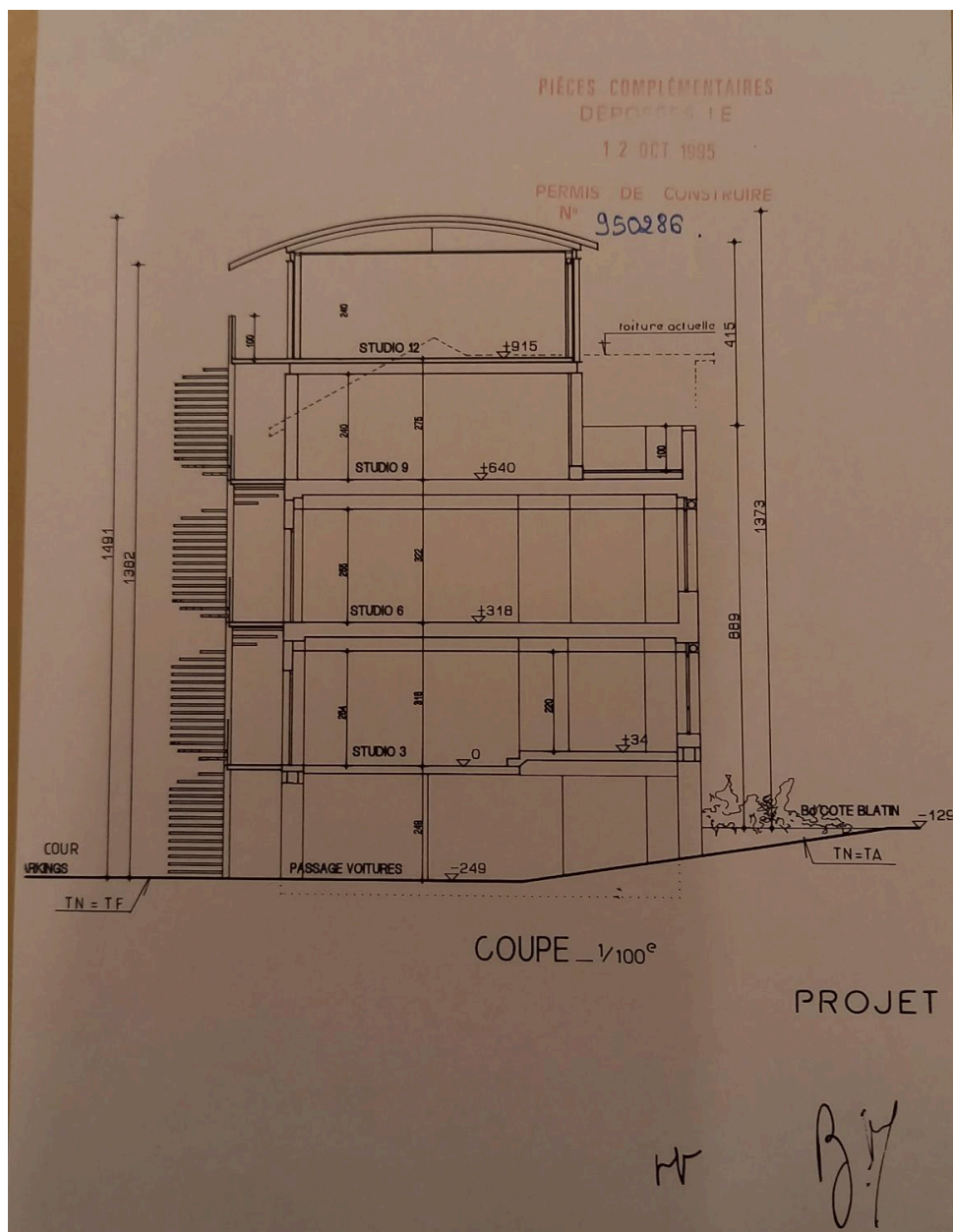
Coupe longitudinale
