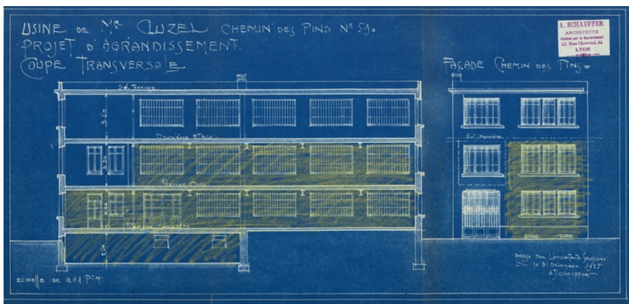
AC Lyon : 344 WP 202 PCA n°0211, coupe transversale de l'usine (surrélévation) de M. Cluzel par M. Schaeffer, 1926
