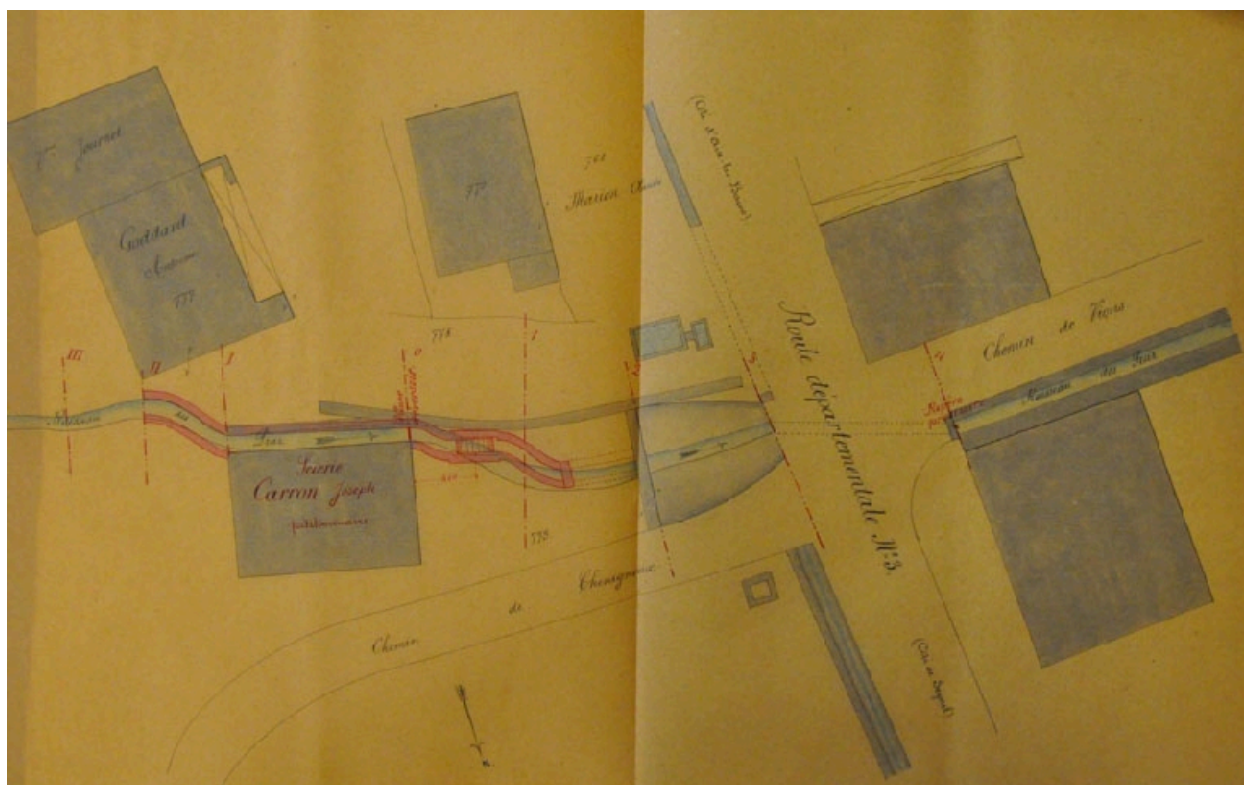
Plan de la prise d'eau de la scierie Carron, 1892. Plan de la prise d'eau de la scierie Carron AD Savoie. 81S33
