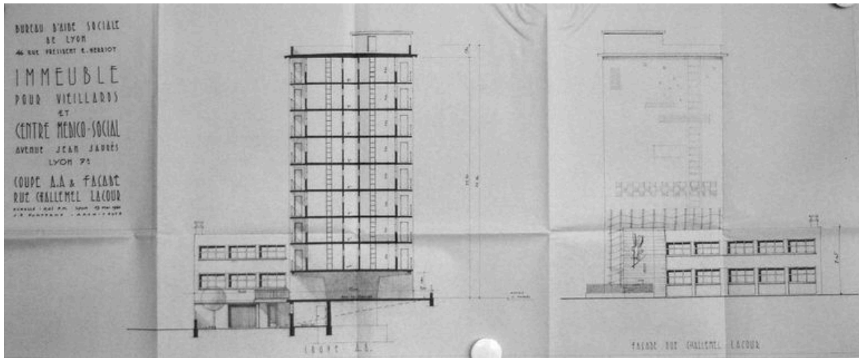
Coupe et façade sur la rue Challemeil-Lacour, immeuble pour vieillards et centre médico-social, 13 mai 1960 par J.P. Fonterme architecte échelle 1/100. (Arch. mun. Lyon)
