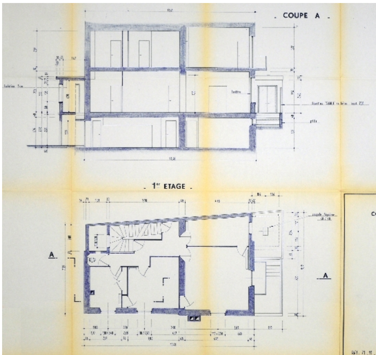
Plan du premier étage et coupe
