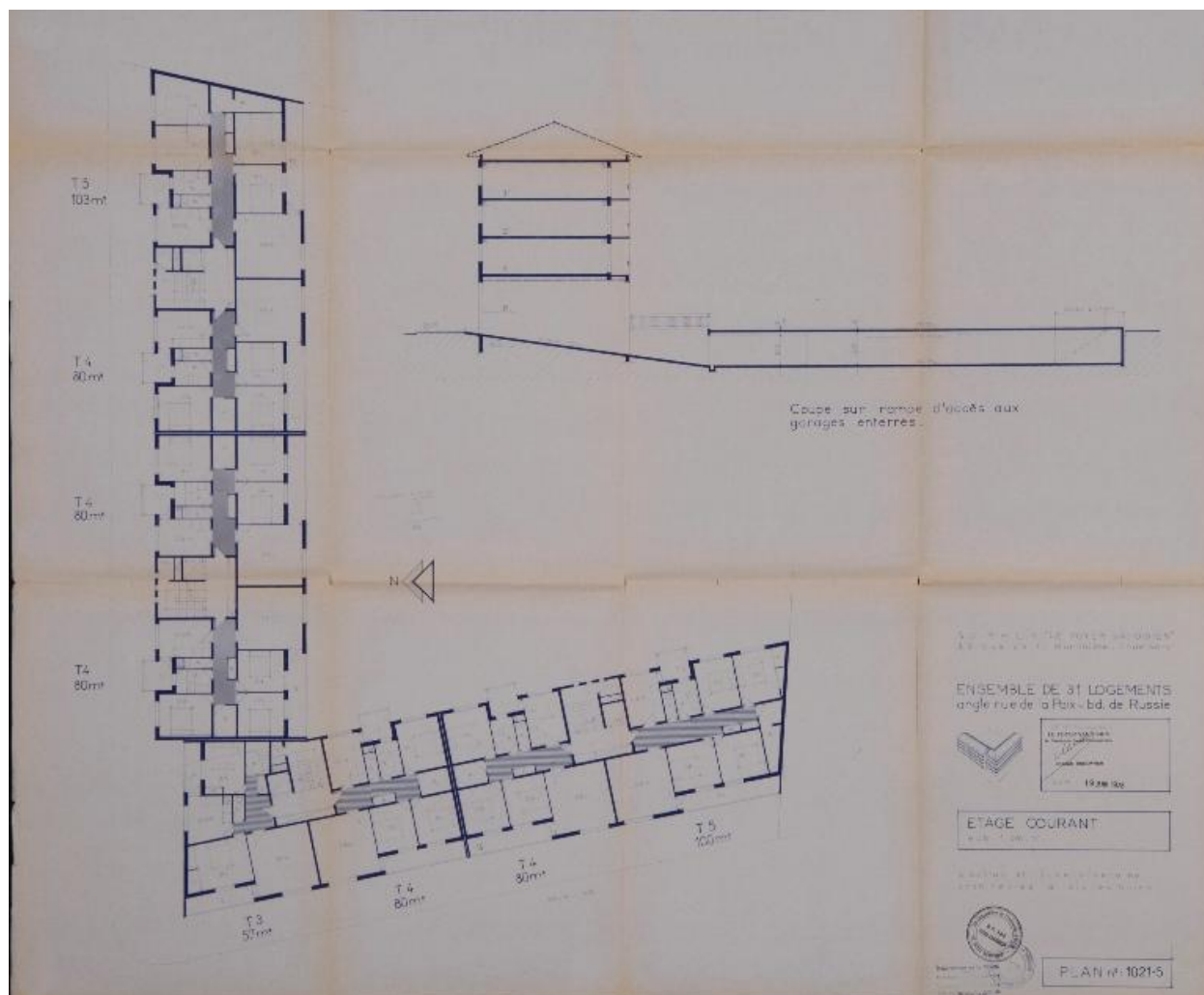
Plan de l'étage courant, 1978
