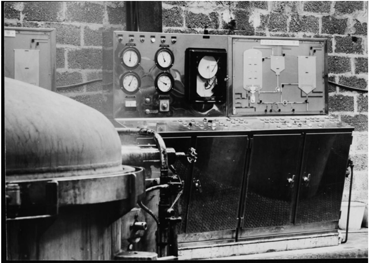
Autoclave de teinture et son appareil de régulation (vers 1960)
