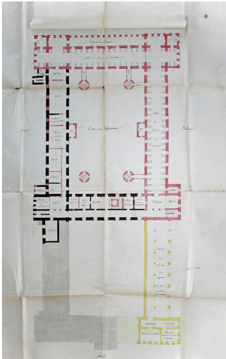
Hôtel-Dieu de Clermont-Ferrand. L'édifice de l'hôtel-Dieu, plan du rez-de-chaussée sur la seconde cour, proposition B (retombe ouverte), 9 mars 1808, Pierre Rousseau architecte.
