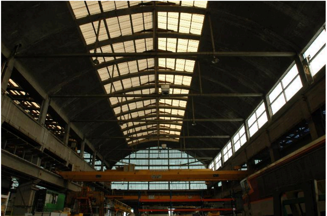
Vue de la charpente métallique des ateliers de réparations
