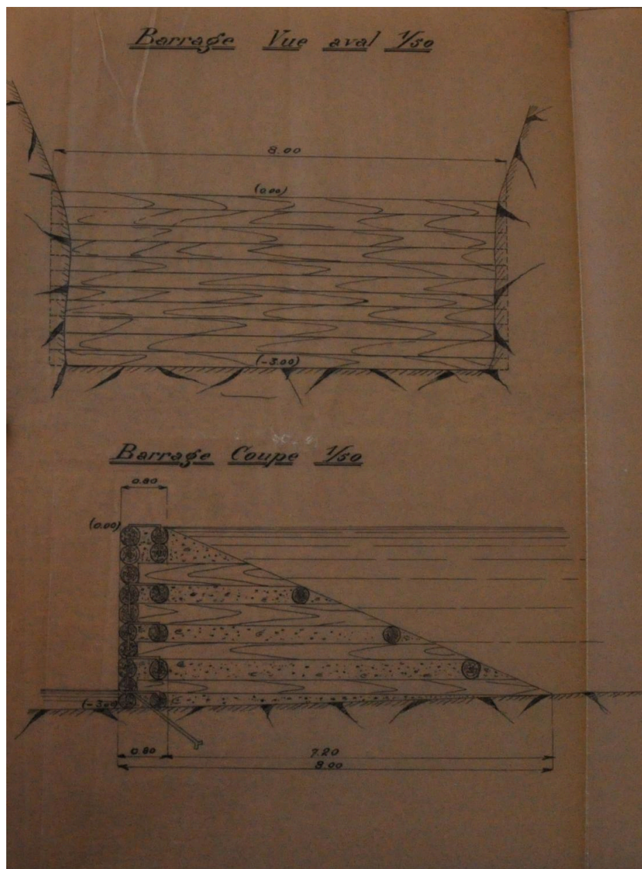
Plan du barrage en bois 1931 (FR.AD073, 82S14).
