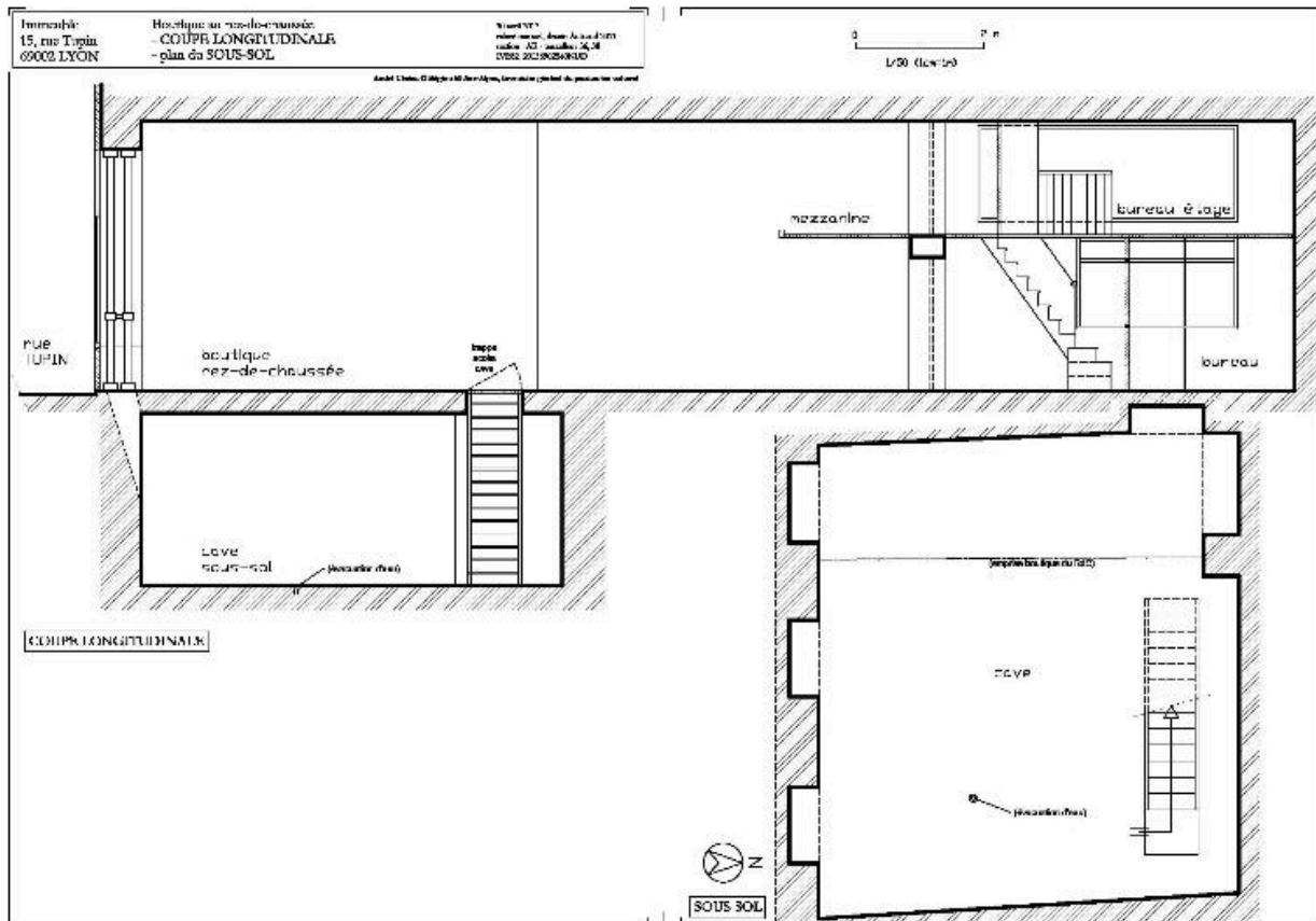
Boutique : plan du sous-sol, coupe longitudinale de l'ensemble
