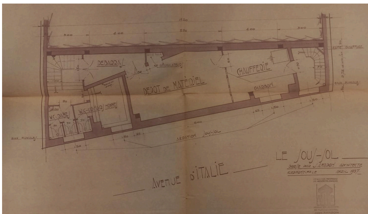
Plan du sous-sol, cinéma le Vox
