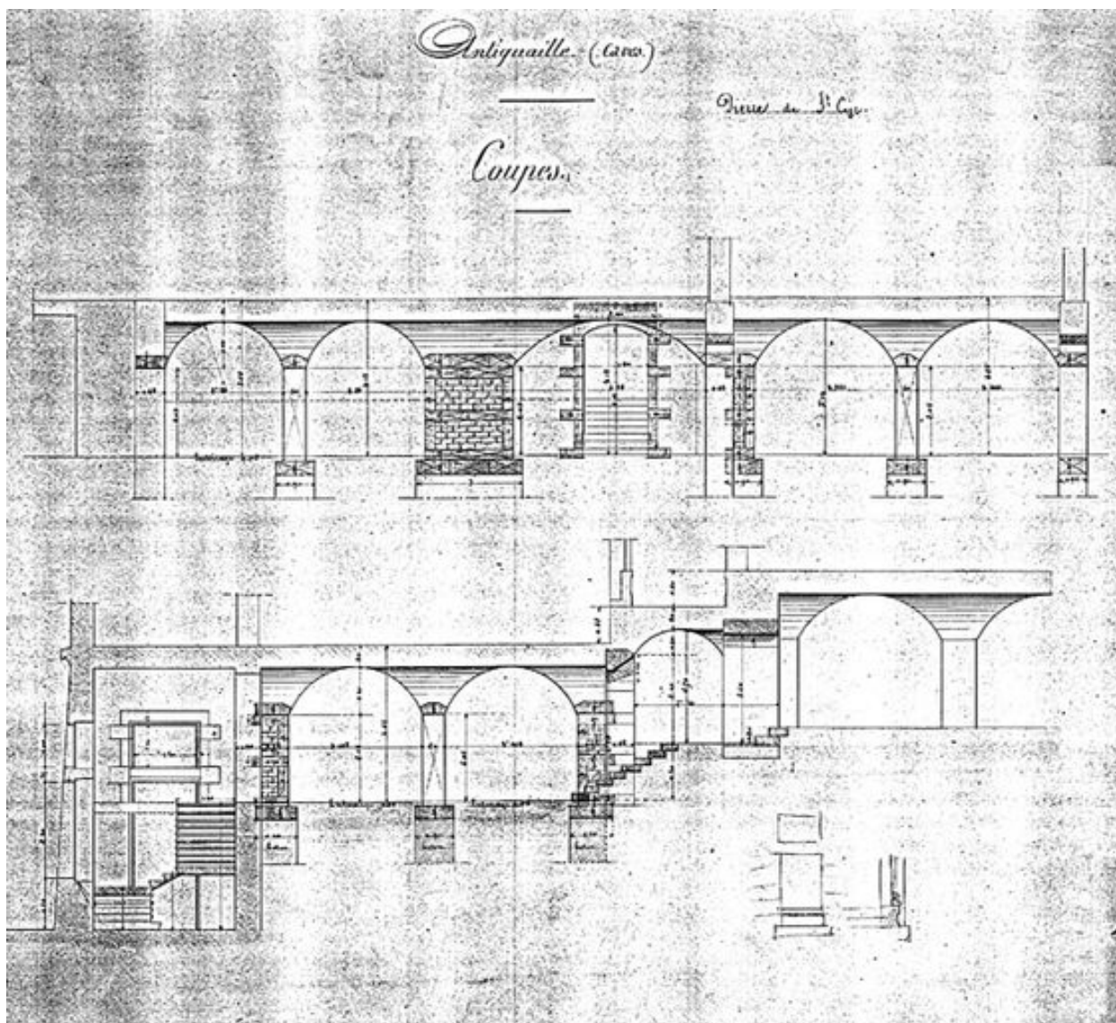
Projet pour la reconstruction des ailes est et sud du cloître, par Paul Pascalon, 1881. 7) Coupes de l'étage de soubassement de l'aile est
