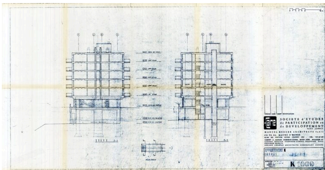
Appartement K. Coupes transversales. Marcel Breuer architecte, 10 septembre 1966 (AC Arâches-la-Frasse)
