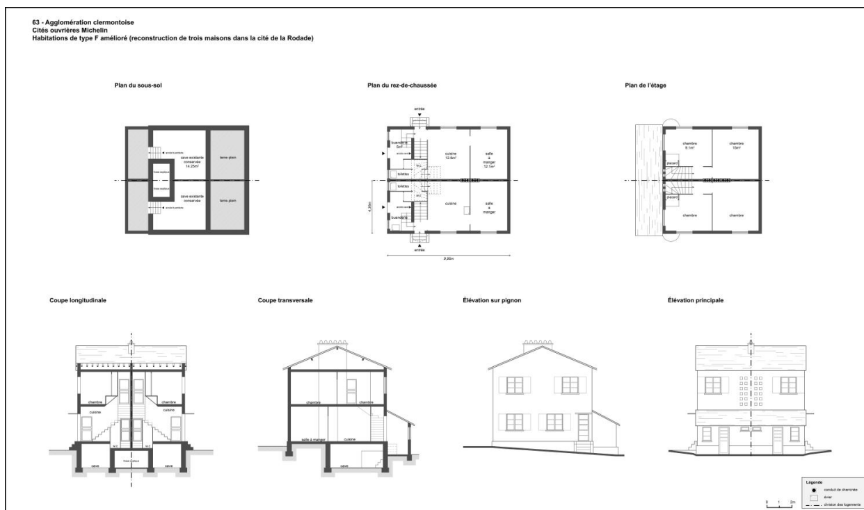
Plans, coupes, façades des habitations de type F amélioré
