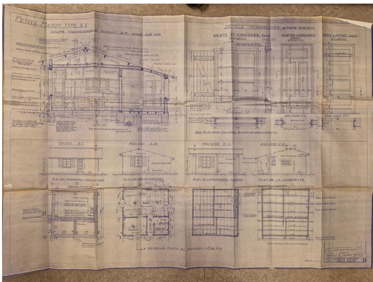
Projet de six maisons individuelles de type X1 : plans, coupes, élévations et détails de menuiseries, 1949.
