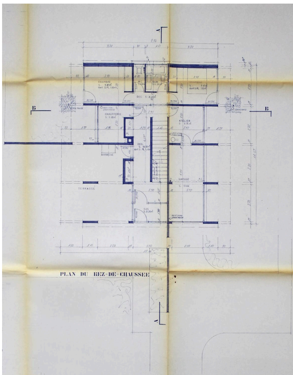
Romagnat, la maison B., plan du rez-de-chaussée, Lucien Ambrosetti et J.-P. Gauer architectes, juin 1969 (archives municipales de Romagnat).
