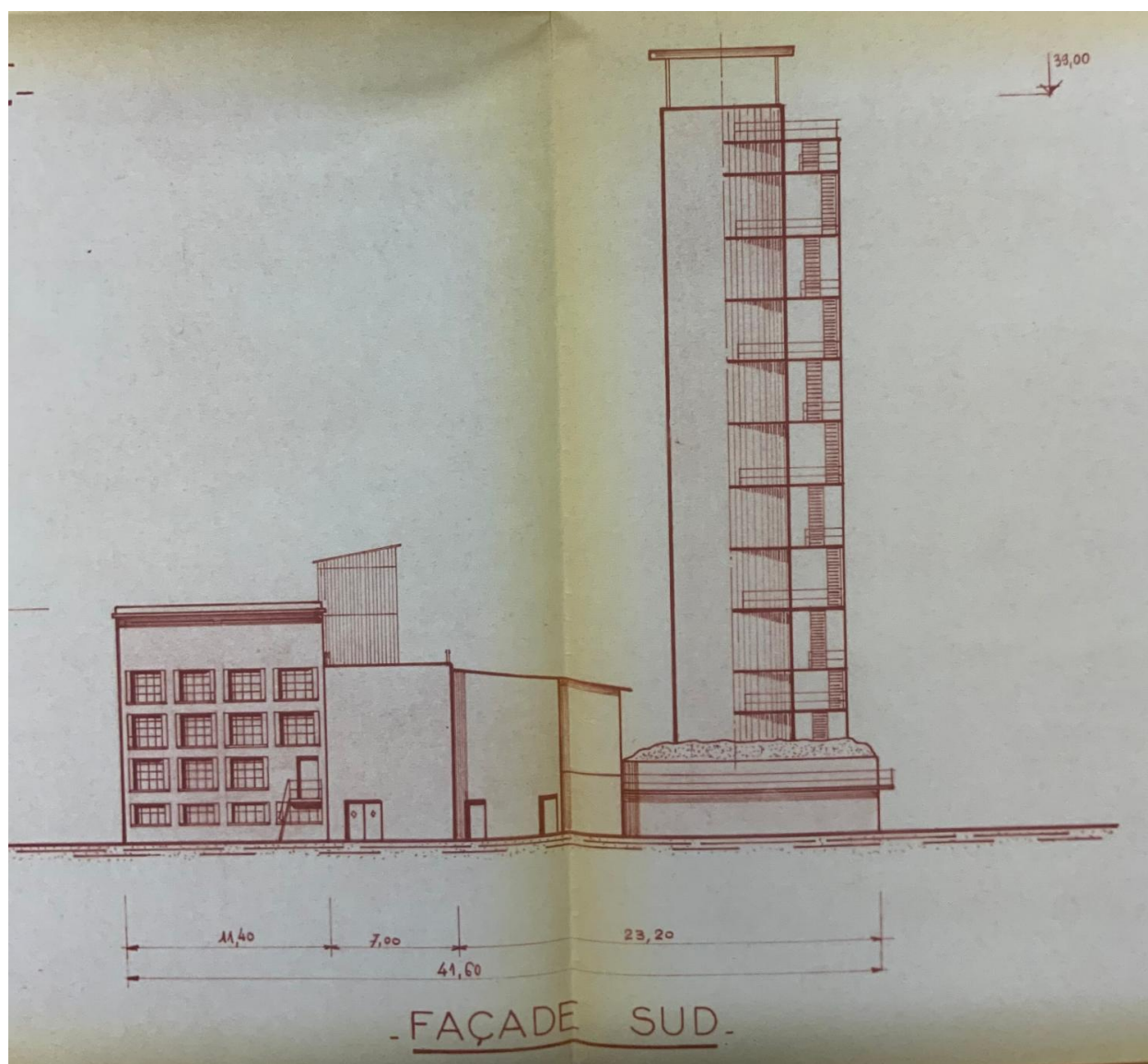
Plan extension façade Sud, tracé par J. Denis, 1971 (AC Pierre-Bénite : 203 – 45)
