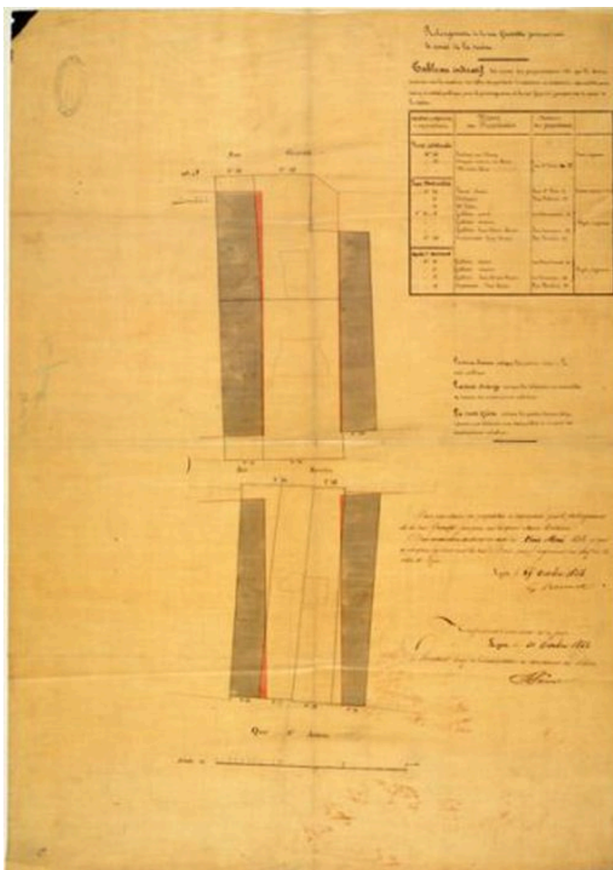
Plan parcellaire des propriétés à exproprier pour le prolongement de la rue Grenette jusques sur le quai Saint-Antoine, par G. Bonnet, 31 octobre 1856. dess. : encre et lavis AM Lyon. 321 WP 111
