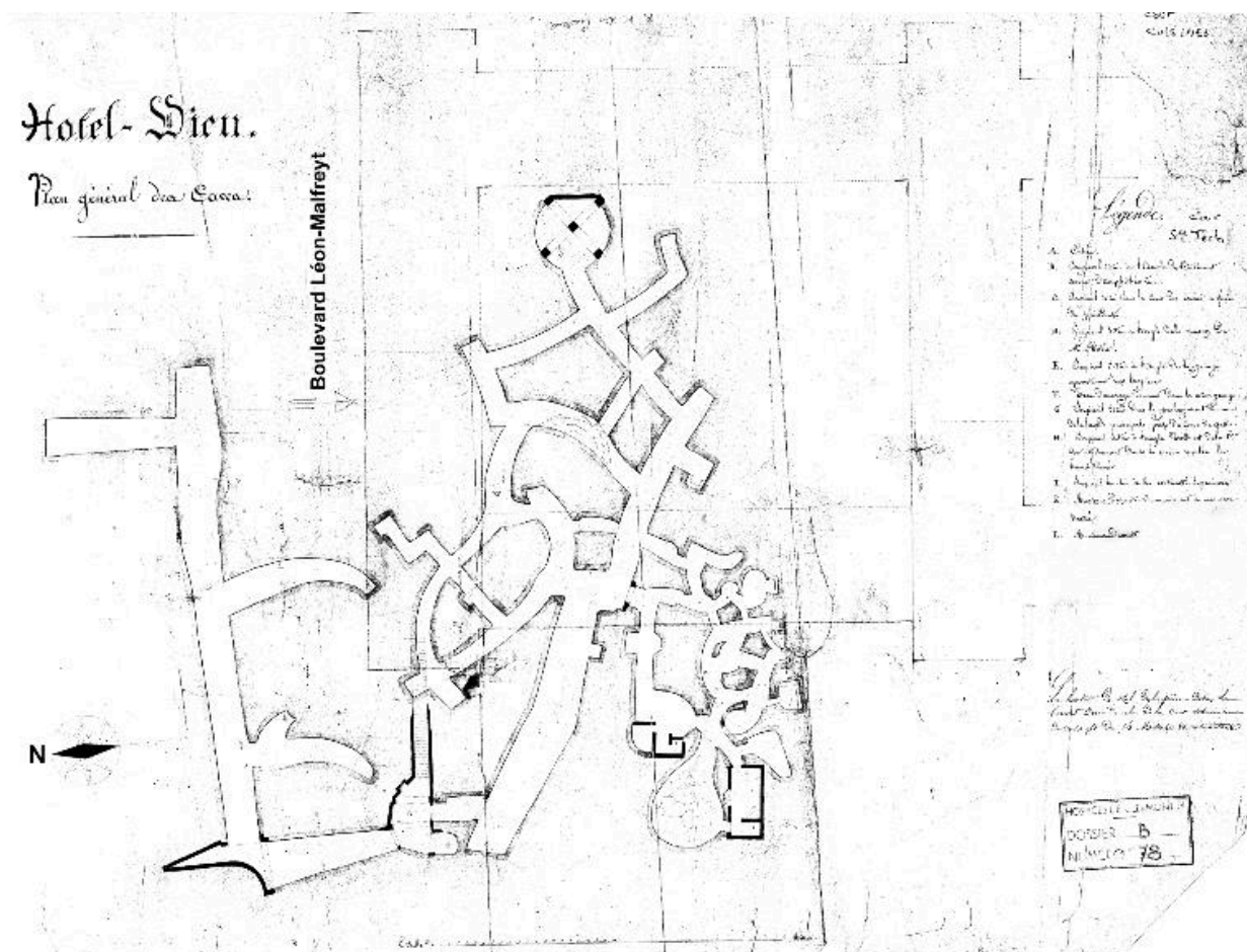
Hôtel-Dieu de Clermont-Ferrand. "Hôtel-Dieu, plan général des caves", levé vers 1830-1850 (l'orientation des galeries est très approximative).
