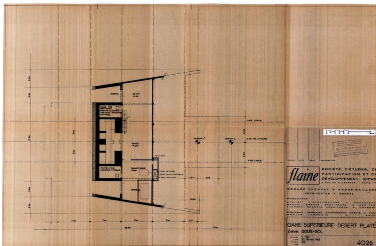
Plan du 2e sous-sol. Gérard Chervaz et André Gaillard architectes, 22 février 1963 (AC Magland)
