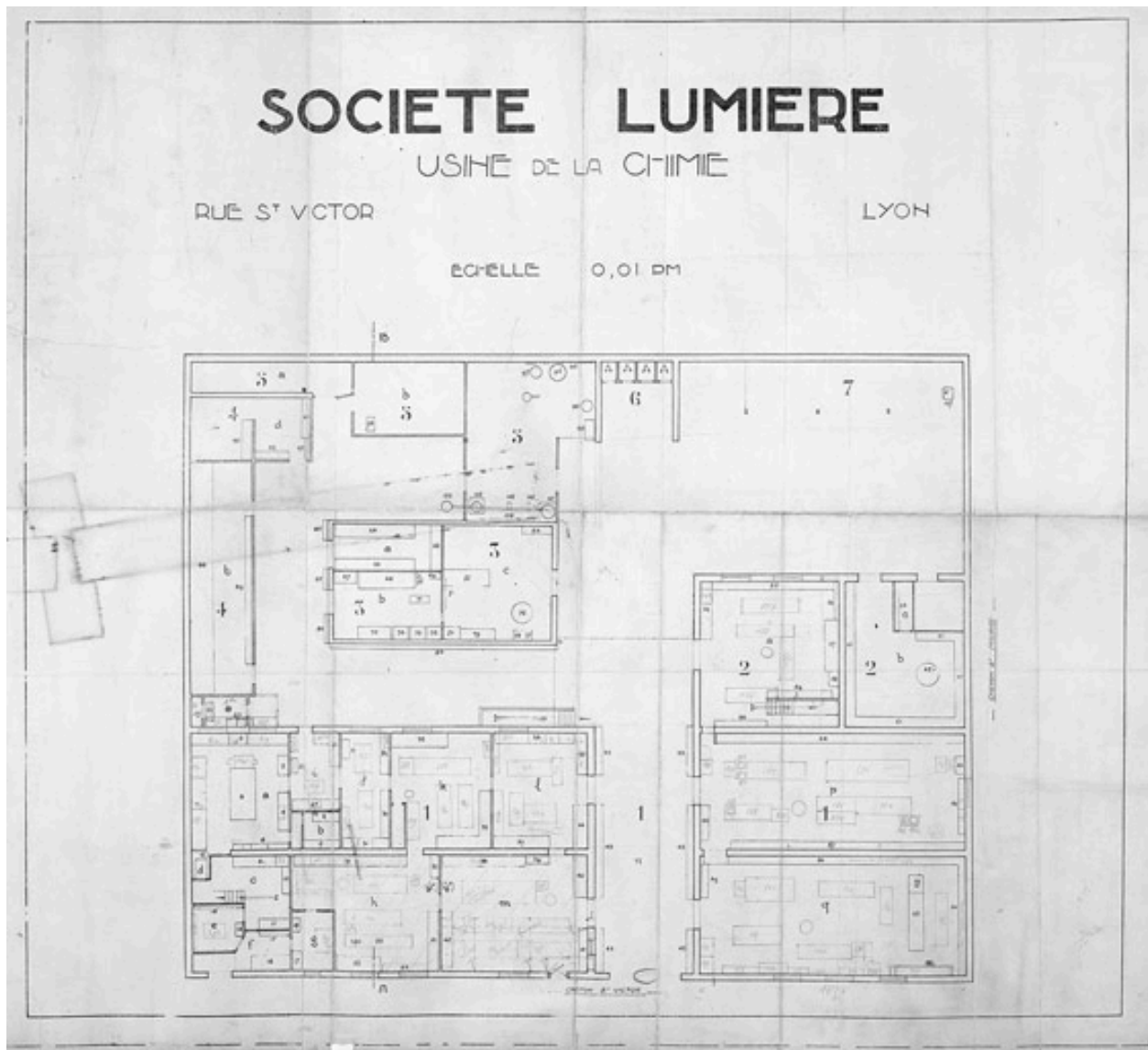
Plan Société Lumière : usine de la chimie
