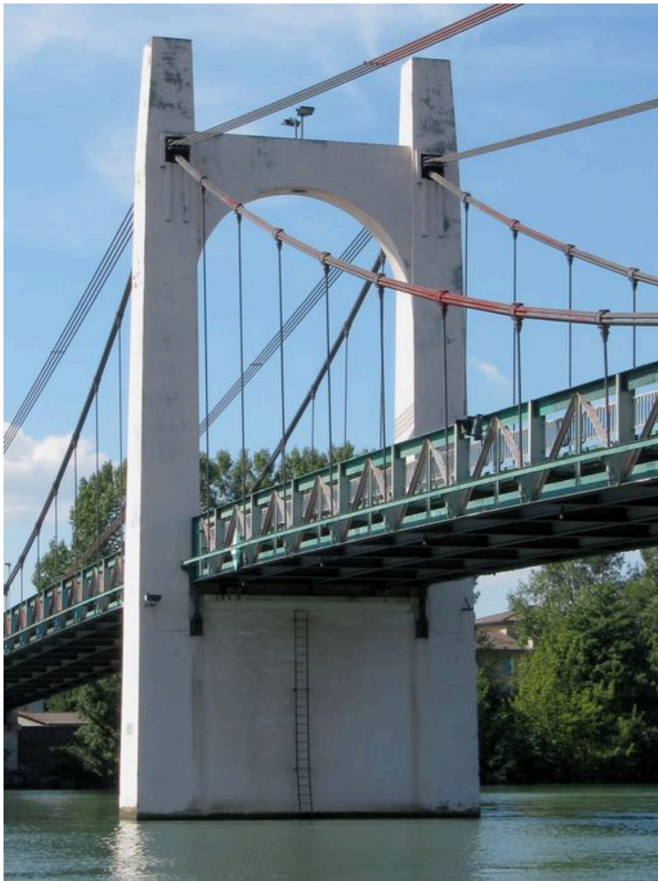
Pylône central, face amont (depuis la rive droite)
